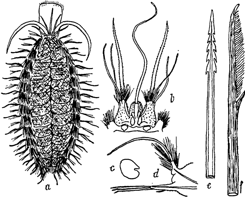
FIG. 12. — Laetmatonice filicornis : a, face dorsale \times 2 ; b, tête; c, 5 e élytre \times 2 ; d, 14 e sétigère (d'après KINBERG); e, f, soie en harpon \times 20 et soie ventrale \times 15 (d'après ROULE).
