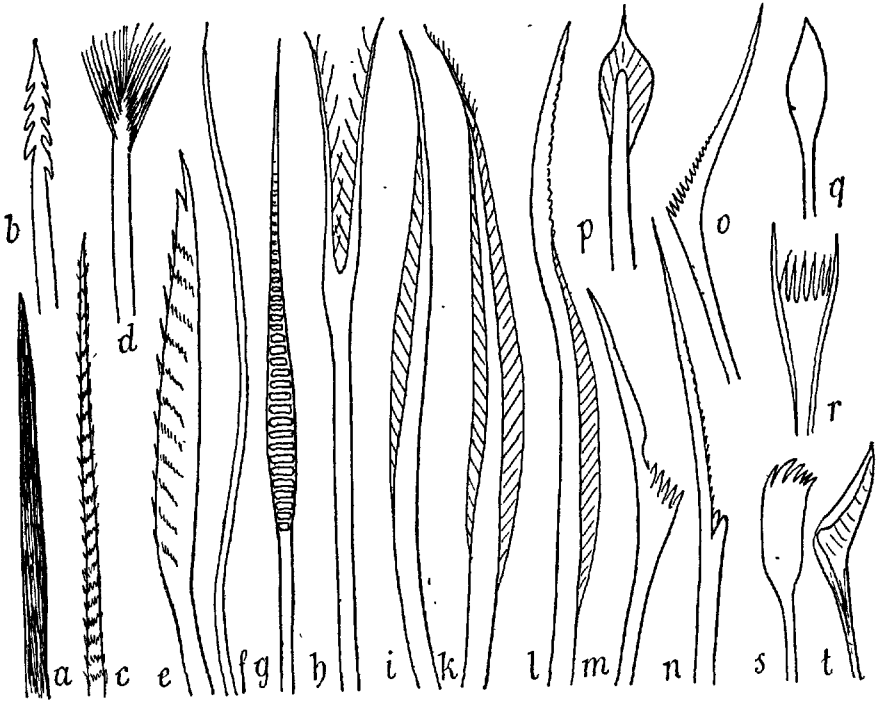
FIG. 4. — Soies simples, grossies de 100 à 200 fois : a, acicule. — b, barbelée d' Hermione . — c, capillaire épineuse. — d, en brosse, de Panthalis ; e, de Lagisca . — f, capillaire lisse. — g, à plaquette, de Nephtys . — h, lyriforme, de Nephtys — i, limbée; — k, bilimbée, d' Amphitrite . — l, d' Apomatus . — m, de Salmacine. — n, de Serpule. — o, géciculée de Serpulien. — p, en palette, de Potamilla . — q, styliiforme, de Chétophtère. — r, pectinée, d'Eunicien. — s, t, palées de Sabellaria .
