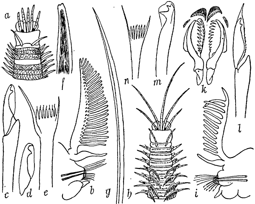
FIG. 158. — Eunice Rousseaui : a, région antérieure grandeur naturelle; b, 32 e pied \times 3 ; c, d, soies composées \times 100 ; e, soie pectinée \times 250 ; f, soie aciculaire \times 150 ; g, soie capillaire limbée \times 150 . — E. vittata : h, région antérieure \times 3 ; i, 40 e pied \times 20 ; k, mâchoire supérieure, grossie; l, soie composée \times 400 ; m, soie aciculaire \times 150 ; n, soie pectinée \times 400 .
