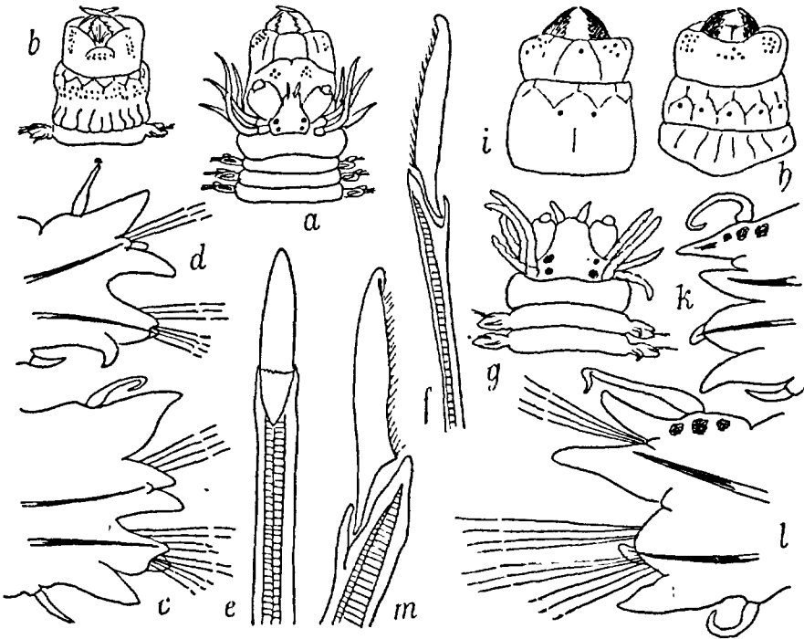
FIG. 133. — Nereis diversicolor : a, b, tête et trompe, grossie; c, 16 e pied \times 20; d, 60 e pied \times 20; e, serpe homopomphe \times 350; f, serpe hétéropomphe \times 350. — N. herguelensis : g, h, i, tête et trompe, grossies (d'après EHLERS); k, 15 e pied \times 40; l, parapode moyen \times 40; m, serpe hétéropomphe \times 350.
