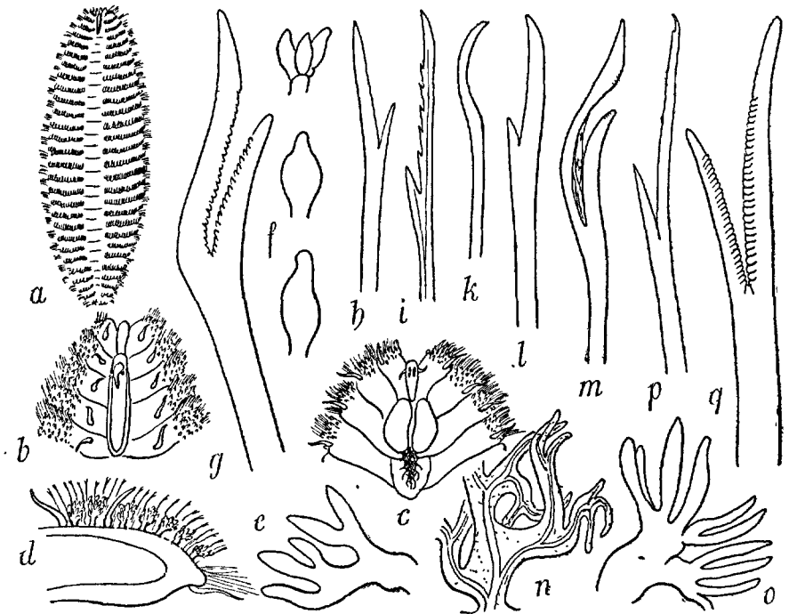
FIG. 49. — Euphosyne foliosa : a, face dorsale, grossie; b, tête, grossie; c, région antérieure, face ventrale; d, parapode, grossi; e, f, diverses variétés de terminaisons branchiales \times 150 ; g, soie dorsale crénelée \times 300 ; h, soie ventrale \times 150 . — E. intermedia : i, soie ventrale \times 160 . — E. myrtosa : k, soie en faux; l, soie bifurquée; m, soie en gueule ( ringent ); n, fragment de branchie (d'après GRAVIER). — E. armadillo o, branchie \times 150 ; p, soie ventrale \times 250 ; q, soie « ringent » \times 250 .
