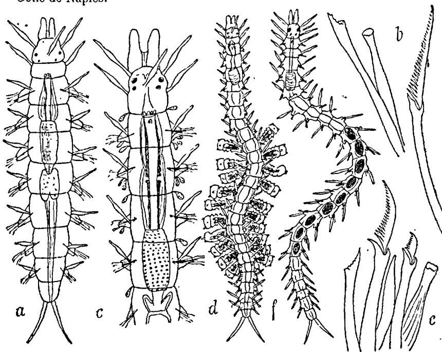
FIG. 141. — Parapionosyllis gestans : a, forme jeune \times 120 ; b, soies \times 1500 . — Par. papillosa : c, région antérieure \times 60 . — Par. elegans : d, avec larves à 3 sétigères \times 20 ; e, soies \times 1500 . — Par. minuta : f, avec œufs \times 23 (d'après PIERANTONI).
