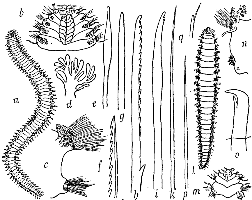
FIG. 47. — Hermodice carunculata : a, grandeur naturelle; b, tête, grossie; c, parapode, grossi; d, branche inférieure; e, soie ventrale hastée \times 150 ; f, extrémité de soie dorsale en harpon \times 300 ; g, extrémité de grosse soie dorsale lisse \times 300 ; h, soie ventrale bifurquée et dentelée \times 300 ; i, soie ventrale \times 300 ; k, soie dorsale capillaire \times 300 . — Hipponoë Gaudichaudi : l, grandeur naturelle; m, tête, grossie; n, parapode, grossi; o, crochet ventral \times 100 ; p, soie dorsale et q, extrémité de soie dorsale bifurquée \times 300 .
