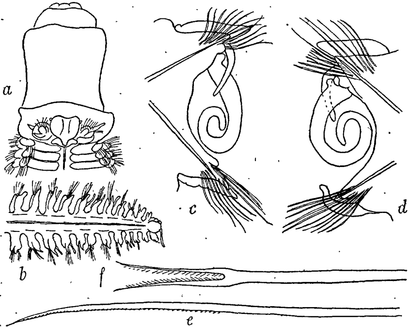
FIG. 147. — Nephthys inermis : a, tête et trompe \times 20 ; b, région postérieure \times 20 ; c, 95 e pied \times 30 ; d, 45 e pied \times 30 ; e, longue soie simple \times 450 ; f, soie lyriforme \times 450 (d'après EHLERS).
