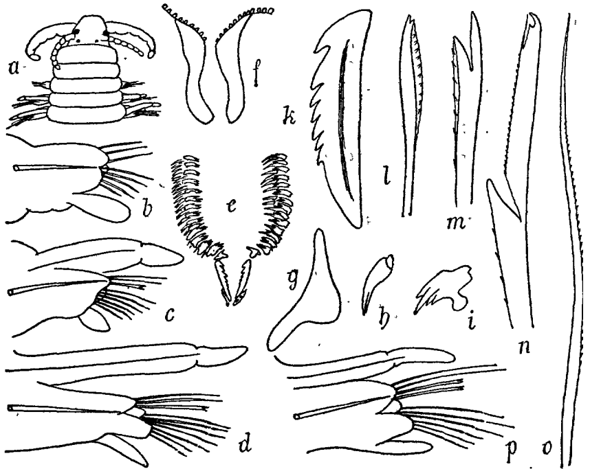
FIG. 178. — Staurocephalus Rudolphii : a, tête, grossie; b, 1 er pied \times 60 ; c, 2 e pied \times 60 ; d, pied moyen \times 60 ; e, mâchoire supérieure, grossie; f, labre \times 40 ; g, pince (mandibule) \times 150 ; h, pièce mandibulaire \times 150 ; i, pièce maxillaire \times 150 ; k, pièce basale de support \times 150 ; l, soie géniculée du 1 er sétigère \times 550 ; m, soie fourchue \times 400 ; n, soie composée \times 550 ; o, soie capillaire \times 500 ; p, parapode moyen d'un spécimen de S c -Vaast \times 60 .
