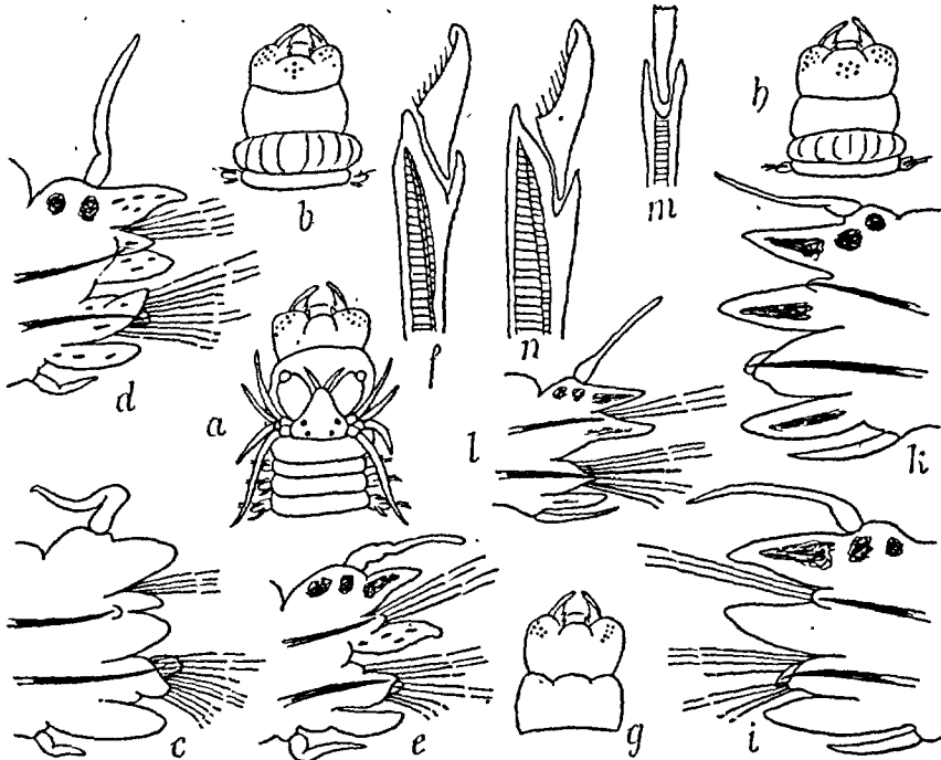
FIG. 136. — Ceratonereis costae : a, b, tête et trompe, grossies; c, d, 11 e et 18 e pied \times 20; e, parapode postérieur \times 20; f, serpe hétérogomphe \times 350. — C. hircinicola : g, h, trompe, face dorsale et face ventrale, grossie; i, k, l, parapodes antérieur, moyen et postérieur \times 20; m, articulation homogomphe de soie en arête inférieure ventrale \times 350; n, serpe hétérogomphe \times 350.
