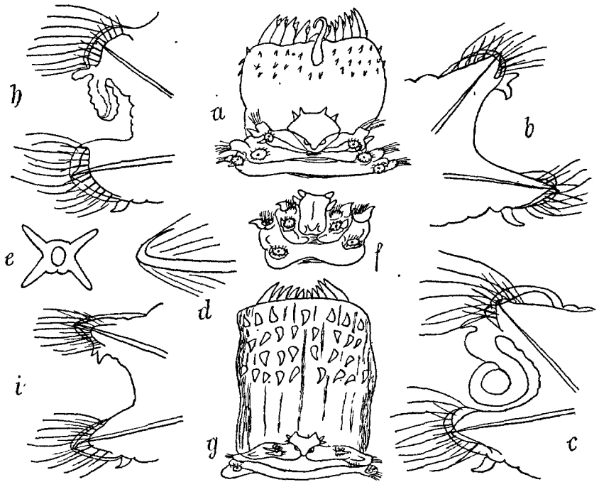
FIG. 146. — Nephthys Hystrixis : a, tête et trompe \times 10 ; b, parapode postérieur \times 12 ; c, parapode moyen \times 12 ; d, pointe de l'acicule \times 150 ; e, section du corps dans la région postérieure. — N. paradoxa : f, prostomium, grossi; g, tête et trompe d'après EHLERS); h, parapode moyen \times 10 ; i, parapode postérieur \times 10 .
