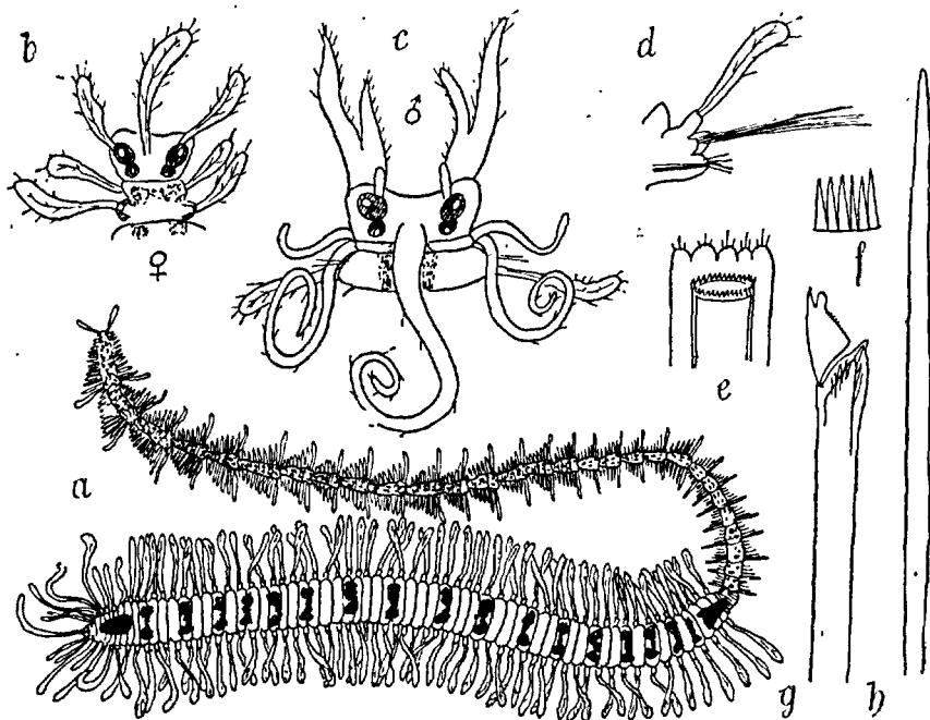
FIG. 124. — Myrianida pinnigera : a, souche suivie de 29 stolons, grossie; b, Sacconereis , région antérieure; c, Polybostrichus , région antérieure; d, parapode d'une forme sexuée; e, trompe (d'après MALAQUIN); f, quelques dents du trépan \times 200 (d'après SAINT-JOSEPH); g, soie composée et h, soie natatoire, très grossie (d'après Mc INTOSH).
