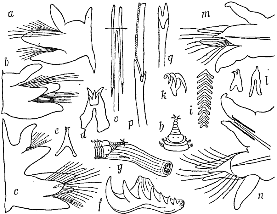
FIG. 154. — Goniada maculata : a, 15° pied \times 50; b, 37° pied \times 45; c, 48° pied \times 35 d, paragnathe en X \times 155; e, paragnathe en Y \times 155 (d'après ARWIDSSON); f, mâchoire très grosse (d'après VOIR); g, tête et trompe \times 10 (d'après EHLERS). — G. emerita : h, tête (d'après MILNE-EDWARDS); i, chevrons; k, mâchoire \times 25 (d'après EHLERS); l, paragnathes \times 60 (d'après SAINT-JOSEPH); m, 50° pied \times 60; n, 140° pied \times 40; o, acicule et soies aciculaires dorsales \times 80; p, q, hampe des soies composées, face et profil \times 350.
