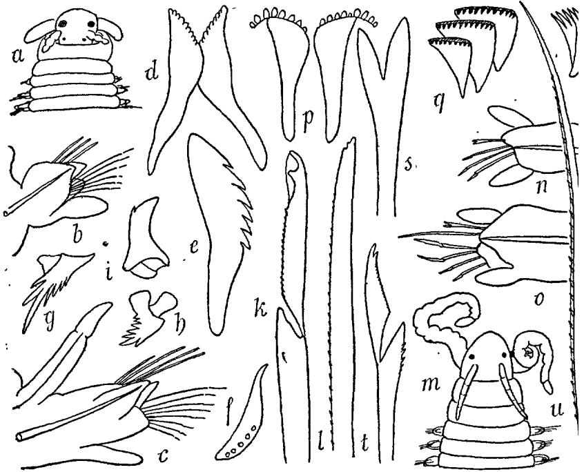
FIG. 177. — Staurocephalus rubrovittatus : a, tête, grossie; b, 1 er pied \times 75; c, p. moyen \times 45; d, labre \times 45; e, grande pièce basale de support, \times 100; f, petite pièce basale de soutien ( sacrum ) \times 100; g, pièce mandibulaire \times 100; h, pièce maxillaire moyenne \times 100; i, pince \times 100; k, soie composée \times 550; l, soie dorsale simple \times 550. — St. Kefersteini : m, région antérieure grossie; n, 1 er pied \times 80; o, p. moyen \times 80; p, labre \times 150; q, pièce de la rangée interne de la mâchoire \times 550; r, pièce externe supérieure \times 400; s, grosse soie en fourche \times 550; t, soie composée \times 550; u, soie capillaire \times 500.
