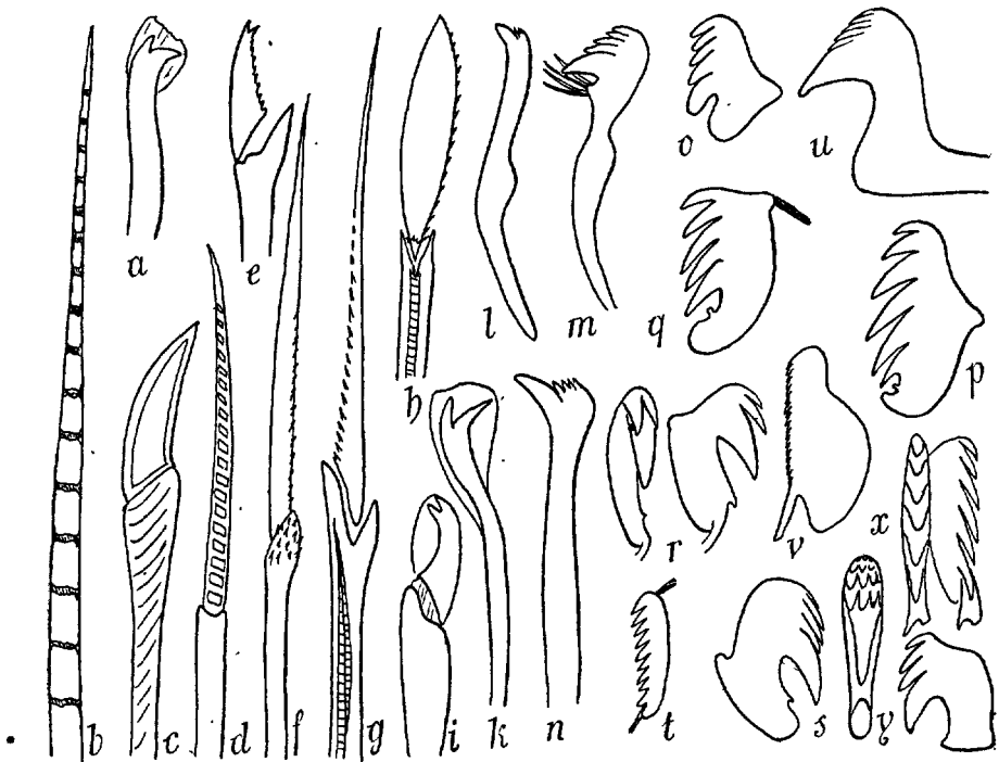
FIG. 5. — Soies : a, aciculaire, d'Eunicien. — b, articulée, de Stylarioides . — c, composée, de Siphonostoma . — d, de Leanira . — e, de Syllis . — f, de Phyllodoce . — g, hétérogomphe, de Nereis . — h, natatoire, d' Heteronereis . — i, en serpe, de Lydidice . — Crochets et uncini grossis de 300 à 400 fois : k, de Polydora . — l, d' Arénicola . — m, de Maldanien. — n, de Trichobranchus . — o, de Serpula . — p, d' Amphiteis . — q, d' Ampharete . — r, de Polymnia , face et profil. — s, d' Amphitrite , face et profil. — t, de Chétoptère. — u, aviculaire de Sabelle. — v, de Protula . — x, de Mercierella . — y, de Chone .
