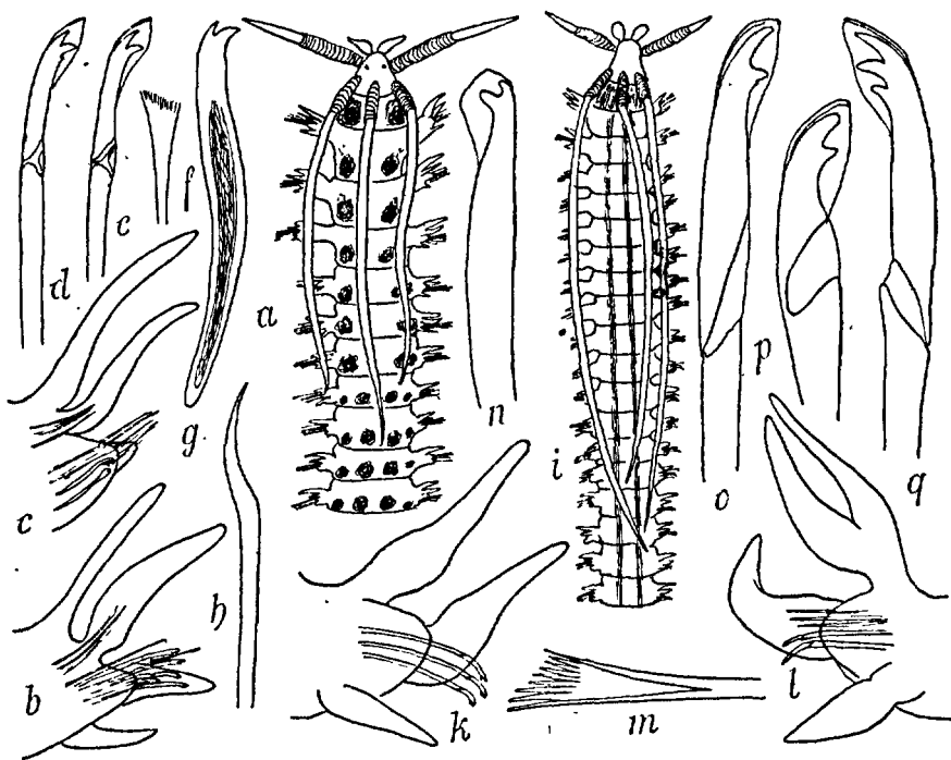
FIG. 167. — Hyalinoccia Fauveli : a, région antérieure \times 4 ; b, 1 er sétigère \times 40 ; c, pied moyen \times 40 ; d, e, soies composées du 1 er sétigère \times 90 ; f, soie pectinée \times 210 ; g, soie aciculaire \times 210 ; h, acicule géniculé \times 210 (d'après RIOJA). — H. bilineata : i, région antérieure \times 20 (d'après RIOJA); k, 1 er sétigère \times 45 ; l, 5 e pied \times 45 ; m, soie pectinée \times 400 ; n, soie aciculaire \times 150 ; o, p, soies composées du 1 er et du 5 e sétigère \times 400 . — VAR. Grubii : q, soie composée \times 400 .
