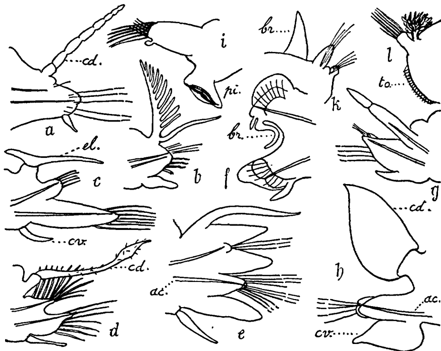
FIG. 3. — Parapodes: a, subbirème, de Podarke pallida . — b, d' Eunice . — c; d, birèmes, élytrigère et cirrigère d'Aphroditien. — e, birème, de Nereis . — f, birème, de Nephthys . — g, sesquirème, de Staurocephalus . — h, unirème, de Phyllococe . — i, distique, d' Amphicteis , rame dorsale et pinnule ventrale. — k, d'Aricien. — l, distique, d'Arénicole. — (ac, acicule; br, branchie; cd, cirre dorsal; cv, cirre ventral; el élytre; pi, pinnule; to, tore uncinigère).
