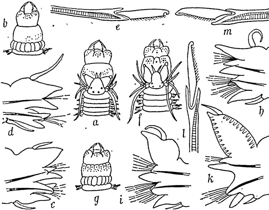
FIG. 135. — Nereis caudata : a, b, tête et trompe, grossies; c, 40 e pied \times 20; d, pied postérieur \times 20; e, serpe hétérogomphe \times 350. — N. succinea : f, g, tête et trompe, grossies; h, 15 e pied \times 20; i, 40 e pied \times 20; k, 60 e pied \times 20; l, serpe homogomphe \times 350; m, serpe hétérogomphe \times 350.
