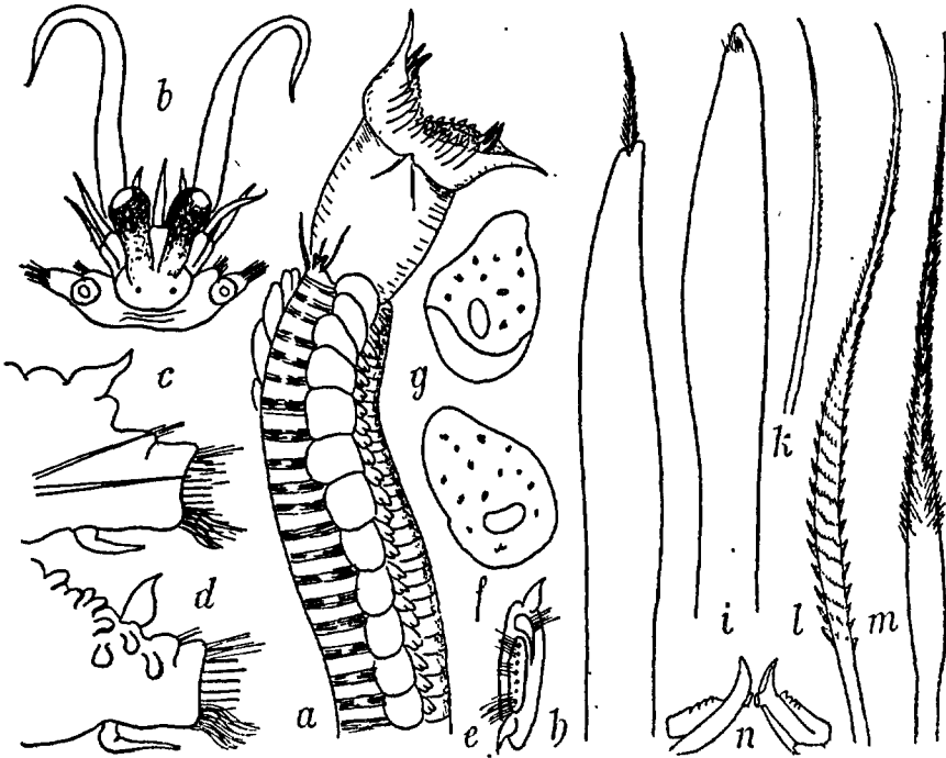
FIG. 37. — Polyodontes maxillosus : a, région antérieure, légèrement réduite, d'après RÉMY-SAINT-LOUP ; b, tête, grossie ; c, parapode antérieur \times 2 ; d, parapode à branchies \times 2 ; e, parapode vu de face \times 2 ; f, g, élytres antérieure et à gousset \times 2 ; h, i, soies aristées \times 100 ; k, soie dorsale \times 100 ; l, soie inférieure ( serrulatae subspirales ) \times 100 ; m, soie ventrale supérieure \times 100 ; n, mâchoire inférieure droite, face interne à gauche, face externe à droite \times 1,5 (d'après PRUVOT et RACOVITZA).
