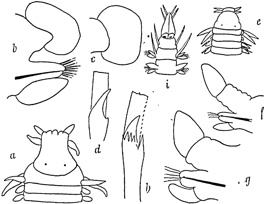
FIG. 63. — Eleone lactea : a, tête \times 8 ; b, 10 e parapode, grossi ; c, cirre dorsal du 5 e sétigère ; d, soie (d'après BERGSTRÖM). — Et. (Mysta) siphonodonta : e, tête, grossie ; f, parapode postérieur ; g, parapode moyen, grossi ; h, soie \times 400 . — Lugia pterophora : i, tête \times 45 (d'après EULERS).
