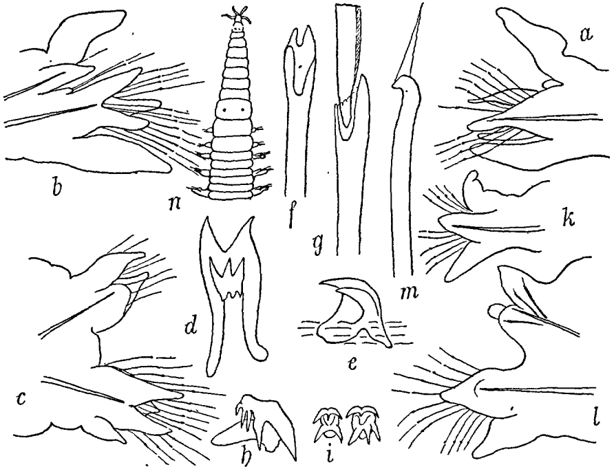
FIG. 155. — Goniada norvegica : a, 20° pied \times 20 ; b, 40° pied \times 20 ; c, pied postérieur \times 20 ; d, paragnathes en X; e, mâchoire (d'après VOIT); f, g, hampe des soies composées, face et profil \times 350 . — Eone Nordmanni : h, mâchoire; i, paragnathes en X (d'après ARWIDSSON); k, pied antérieur \times 30 ; l, pied postérieur \times 30 ; m, soie aciculaire dorsale \times 350 ; n, région antérieure grossie.
