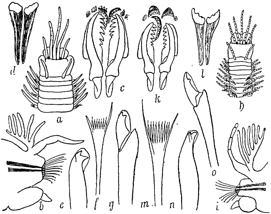
FIG. 157. Eunice floridana : a, région antérieure \times 2 ; b, 31 e pied \times 12 ; c, mâchoire supérieure, grossie; d, labre, grossi; e, soie aciculaire \times 120 ; f, soie pectinée \times 300 ; g, soie composée \times 150 . — E. torquata : h, région antérieure \times 3 ; i, parapode antérieur \times 12 ; k, mâchoire supérieure, grossie; l, labre, grossi; m, soie pectinée \times 400 ; n, soie aciculaire \times 120 ; o, soie composée \times 250 .
