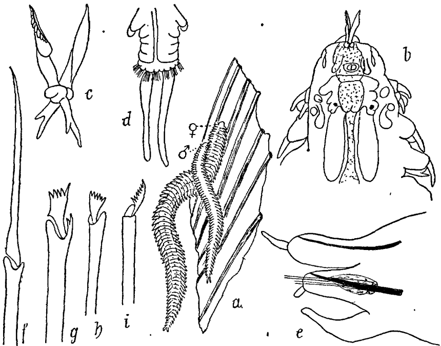
FIG. 181. — Ichthyotomus sanguinarius : a, ♂ et ♀ fixés sur la nageoire de Myrus vulgaris \times 6 ; b, région antérieure, le cerveau, les glandes hémophiles et le pharynx sont vus par transparence; c, les deux stylets de la mâchoire; d, pygidium; e, parapode; f, g, h, i, soies, très grossies (d'après ERSIG).
