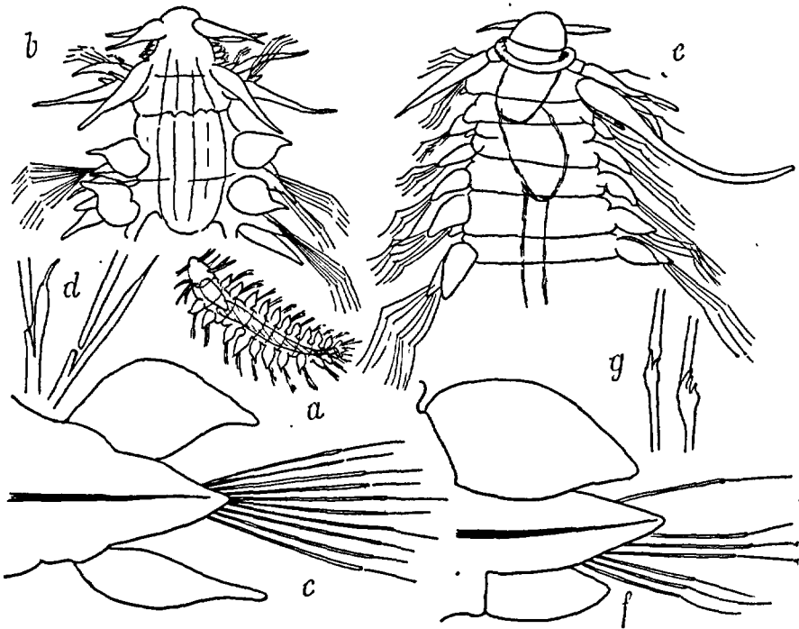
FIG. 74. — Maupasia caeca : a, face dorsale \times 8 ; b, extrémité antérieure \times 25 (d'après VIGIER); c, parapode (d'après BERGSTROM). — VAR. atlantica : d, soies composées (d'après SOUTHERN). — M. magna : e, région antérieure, grossie; f, parapode; g, soies (d'après SOUTHERN).
