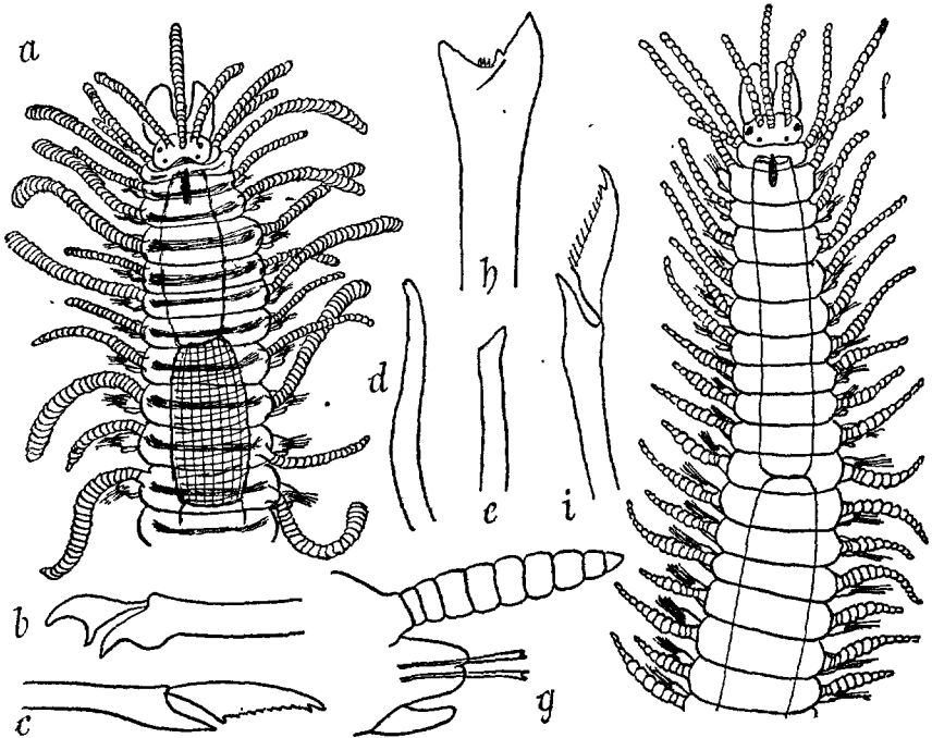
FIG. 96. — Syllis Krohnii : a, région antérieure, grossie; b, soie composée moyenne \times 500 ; c, soie antérieure \times 500 ; d, soie ventrale simple \times 500 ; e, acicule \times 500 . — S. gracilis : f, région antérieure, grossie; g, parapode; h, grosse soie simple \times 500 ; i, soie composée \times 500 .
