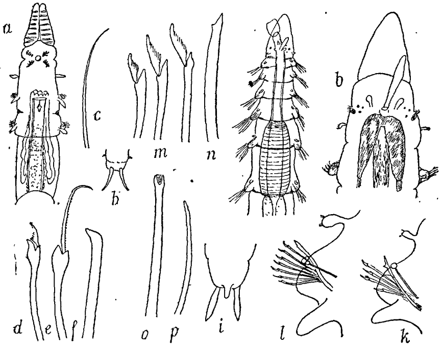
FIG. 118. — Spermophilis torulosa : a, région antérieure \times 20 (d'après CLAPARÈDE); b, cirres anaux; c, soie subulée; d, e, soies composées; f, acicule (d'après SOULIER). — Exogone hebes : g, région antérieure \times 40 (d'après MESNIL); h, tête \times 150 ; i, pygidium \times 100 ; k, parapode antérieur \times 250 ; l, parapode postérieur \times 300 (d'après SOUTHERN); m, soies composées \times 750 ; n, soie dorsale simple \times 750 ; o, acicule \times 750 ; p, acicule excentrique \times 750 (d'après MESNIL).
