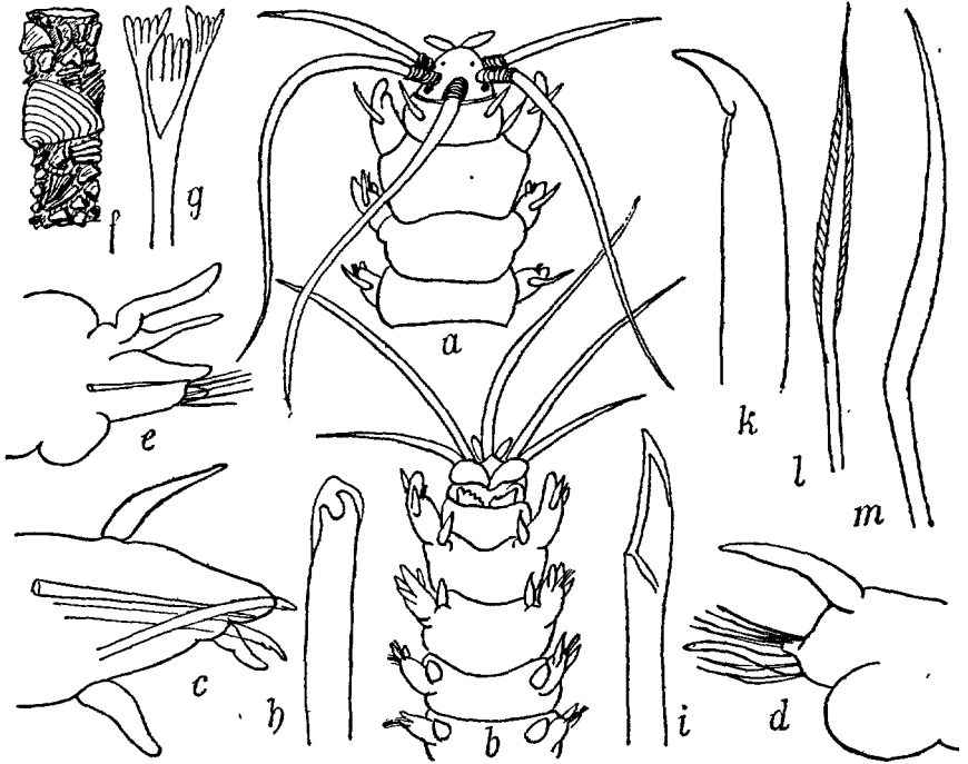
FIG. 164. Onuphis conchylega : a, b, région antérieure, face dorsale et face ventrale \times 4 ; c, 1 er pied \times 30 ; d, 8 e pied \times 30 ; e, 20 e pied \times 30 ; f, tube, grandeur naturelle; g, soie pectinée \times 400 ; h, soie aciculaire \times 150 ; i, soie pseudocomposée \times 150 ; k, soie à crochet du 2 e sétigère \times 100 ; l, soie capillaire limbée \times 100 ; m, soie capillaire \times 100 .
