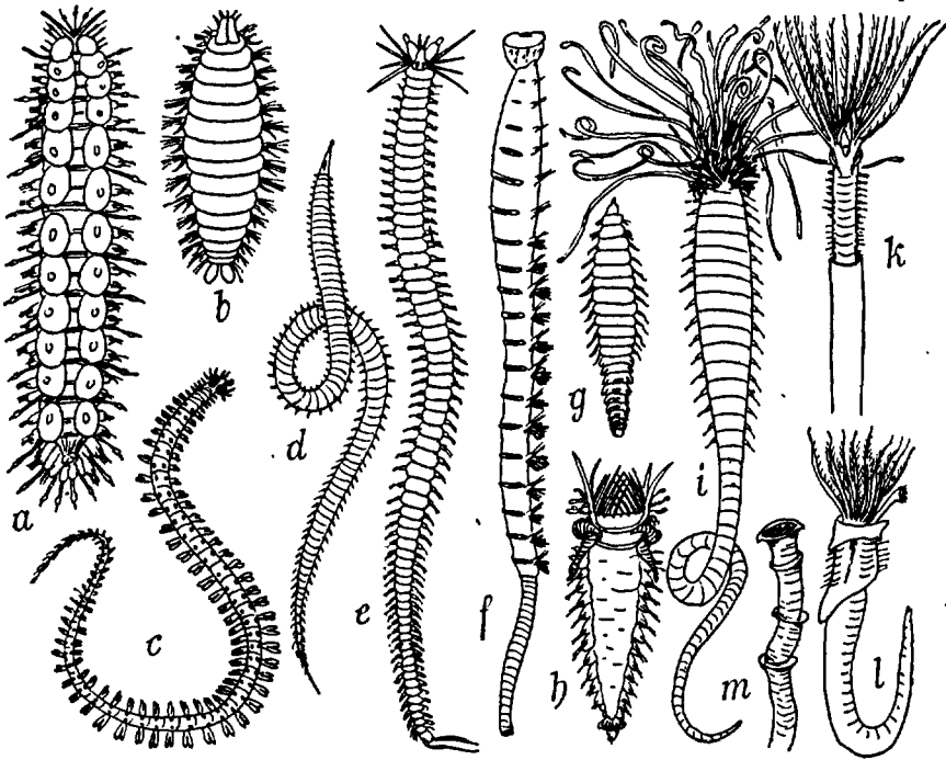
FIG. 1. — a, Lepidonotus clava . — b, Notopygos megalops . — c, Callizona Angelini . — d, Glycère . — e, Perinereis cultrifera . — f, Arenicola marina . — g, Traviisia œstroïdes . — h, Lagis Koreni . — i, Térébelle. — k, Sabelle. — l, Mercierella enigmatica et son tube m, grossis. Toutes les autres figures sont environ de grandeur naturelle.
