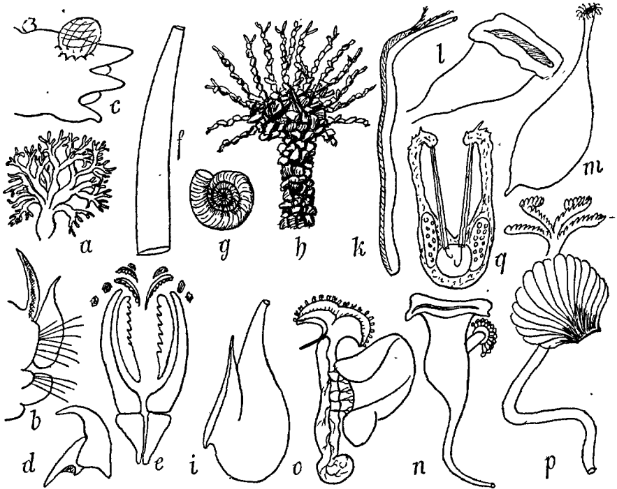
FIG. 6. — a, branchie] de Térébelle. — b, de Spionidien avec branchie dressée. — c, pied de Glycera gigantea avec branchie coelomique rétractile. — d, mâchoire de Glycère. — e, mâchoires d'Eunicien. — f, tube de Pectinaire. — g, tube de Spirorbe. — h, tube de Lanice conchilega . — Néphridies : i, d' Amphicteis . — k, d' Ampharete . — l, d'Eunicien. — m, de Nereis . — n, d' Eulalia (d'après FAGE). — o, d' Arenicola ecaudata avec gonade ♂. — p, de Nephthys et solénocytes q (d'après GOODRICH).
